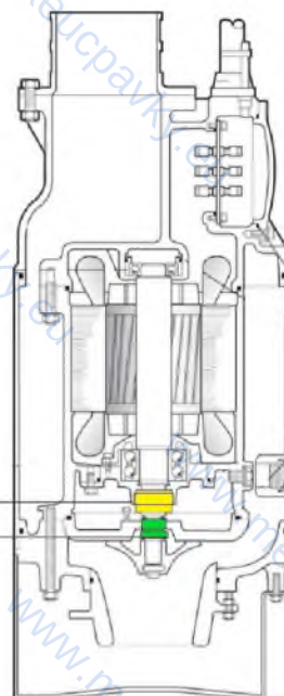
HORNÍ (vnitřní) ucpávka
